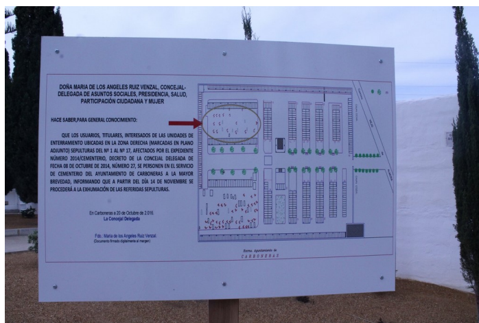
Plano del Cementerio de San José©
